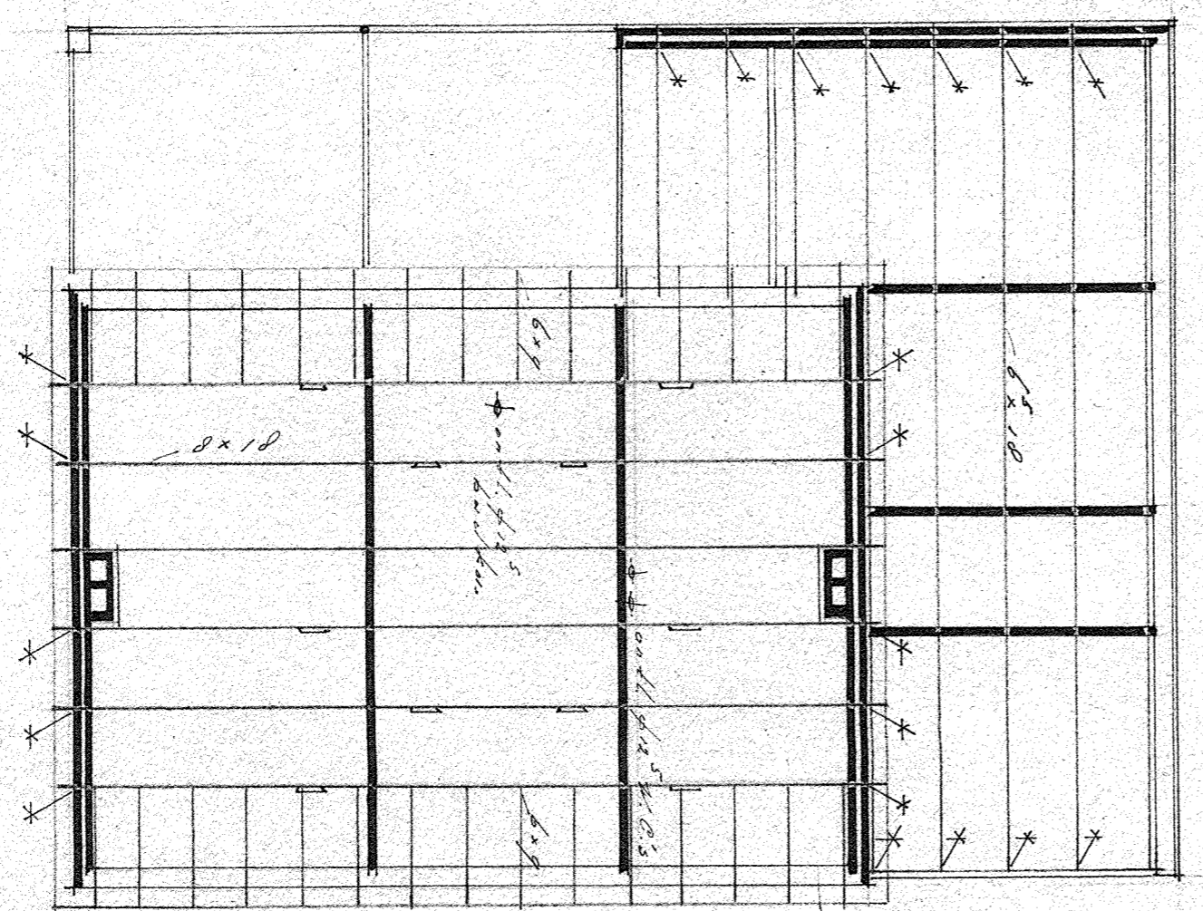
kappplan
