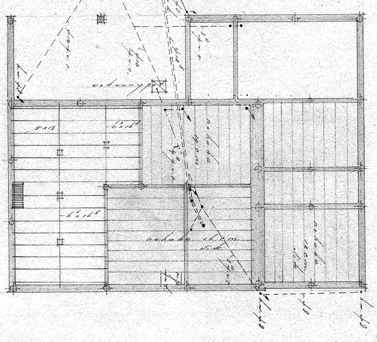
fund.-riol.-vloerl. plan
