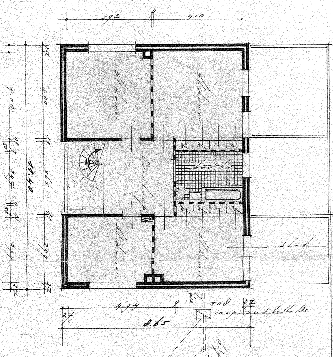
verdieping
