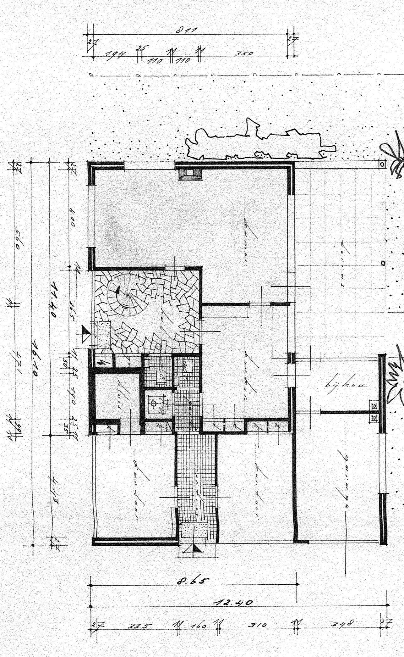
begane grond
